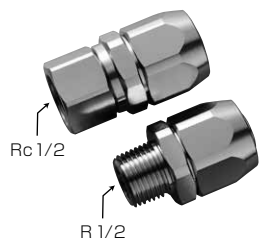
13mm 自在金具セット
