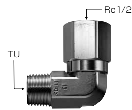
G513 PT1/2メネジL型自在アダプター
