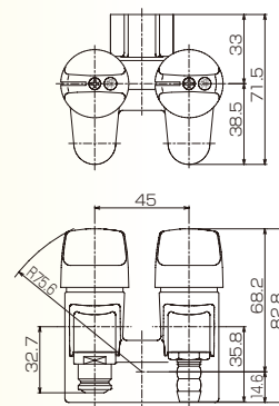
LB二口ペアON・OFFヒューズガス栓 G025-12(R, L)
