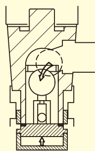
半開(中間開栓)時
