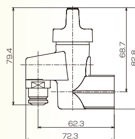
LB一口コンセントON・OFFヒューズガス栓 G015A-12
