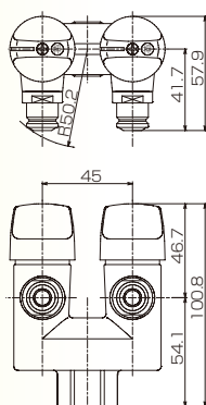
LA二口コンセントON・OFFヒューズガス栓 G023A-12
