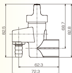
LB一口ON・OFFヒューズガス栓 G015-12
