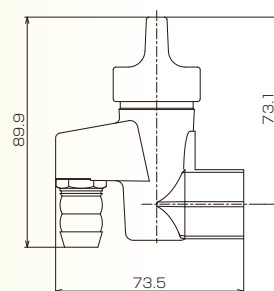
LB一口ON・OFFヒューズガス栓 G015-21
