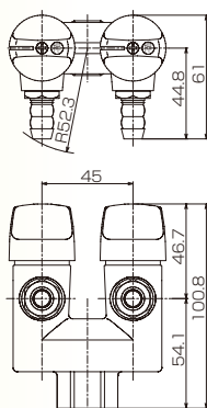
LA二口コンセントON・OFFヒューズガス栓 G023A-12
