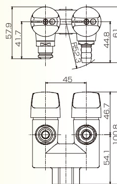
LA二口ペアON・OFFヒューズガス栓 G023-12(R, L)
