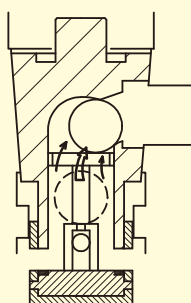
ヒューズ作動時
