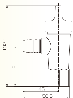
LA一口ON・OFFヒューズガス栓 G013-21
